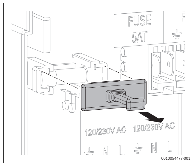
Afb. 32 Zekering vervangen
