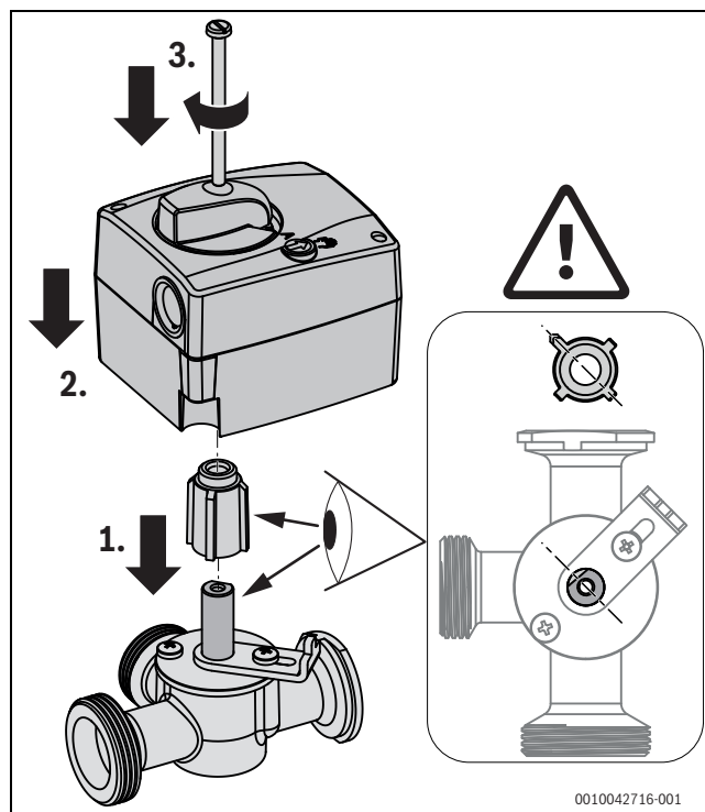
Afb. 35 Mengkraanmotor monteren
