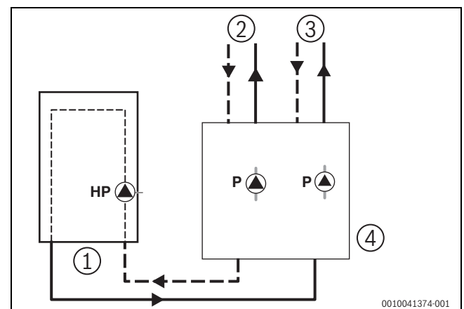
Afb. 3 Overzicht
