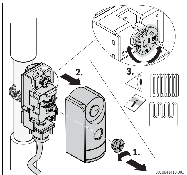
Afb. 20 Temperatuur instellen
