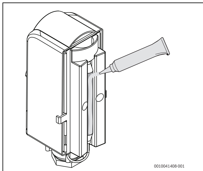
Afb. 18 Warmtegeleidingspasta opbrengen
