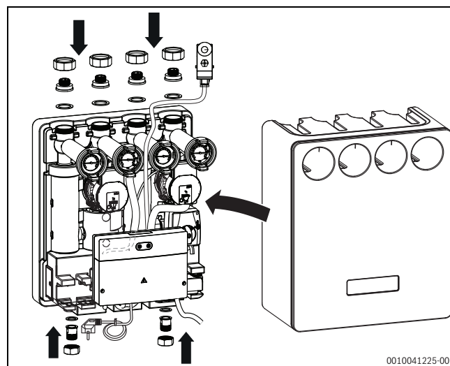
Afb. 16 Montage isolatie
