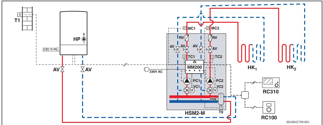
Afb. 2 Toepassingsvoorbeeld HSM2-M 20/7 MM200
