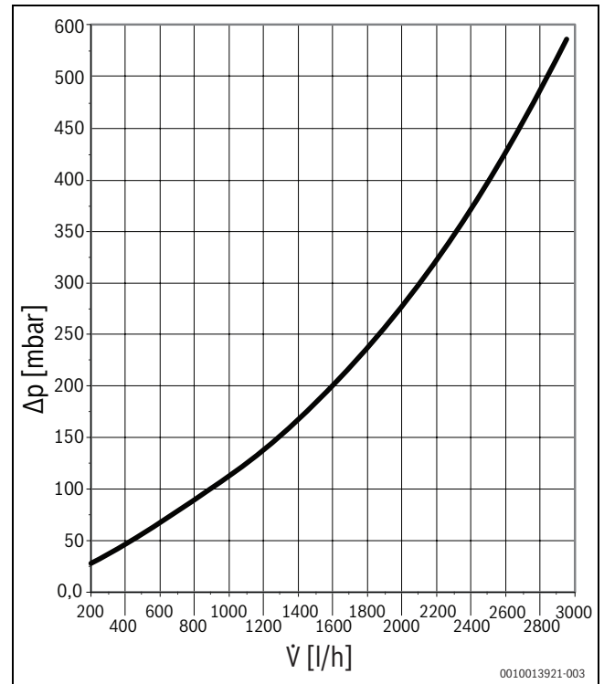
Afb. 11 Drukverliesdiagram gemengd cv-circuit
