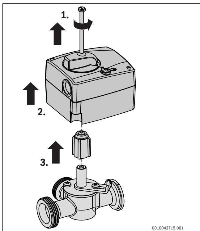
Afb. 34 Mengkraanmotor afnemen
