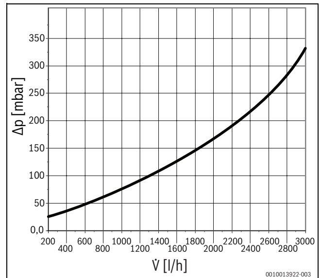
Afb. 12 Drukverliesdiagram ongemengd cv-circuit
