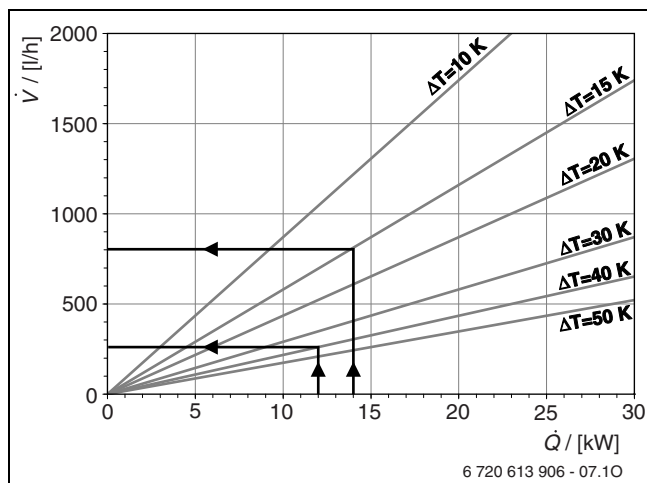
Afb. 4 Debiet-verwarmingsvermogen
