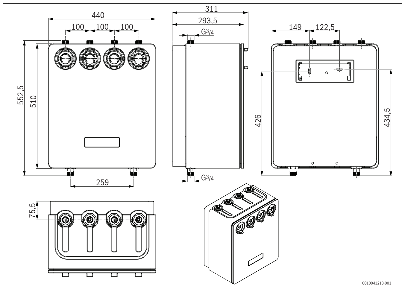
Afb. 10 Afmetingen en aansluitingen (afmetingen in mm)
