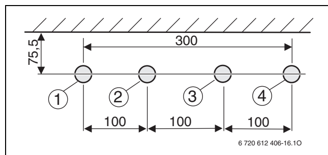
Afb. 17 Afmetingen voor bouwzijdige installatie aansluitingen
