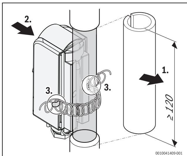
Afb. 19 Temperatuurbewaking monteren
