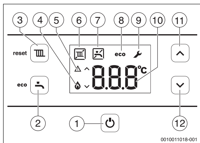
Fig. 5 Messages d'écran
