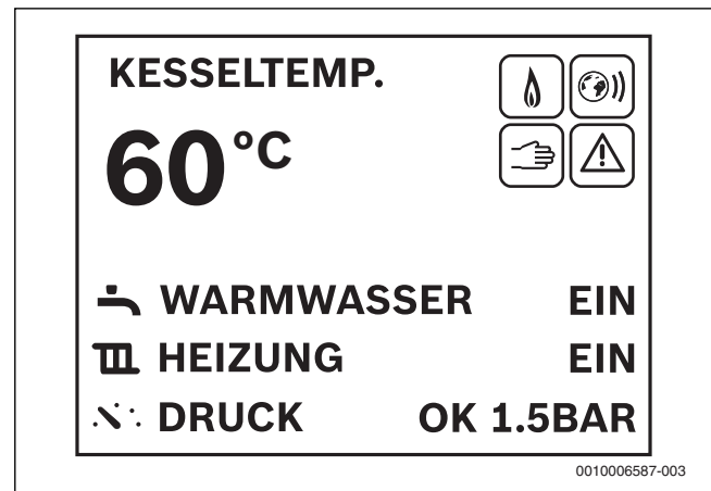
Bild 6 Standardanzeige
