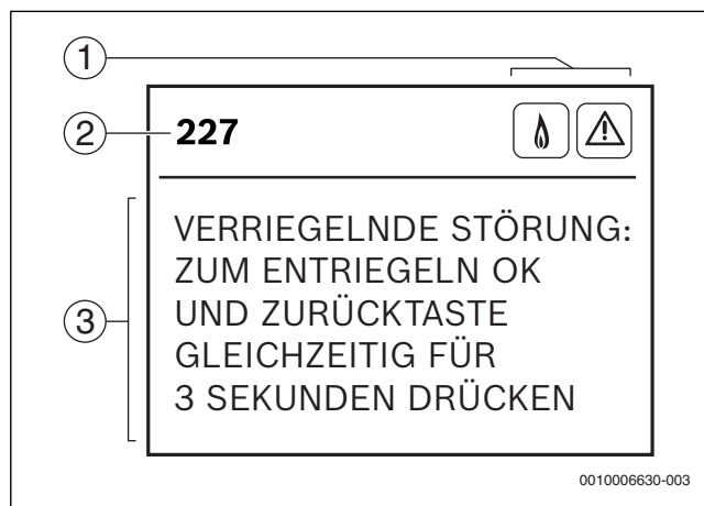
Bild 9 Störungsmenü
