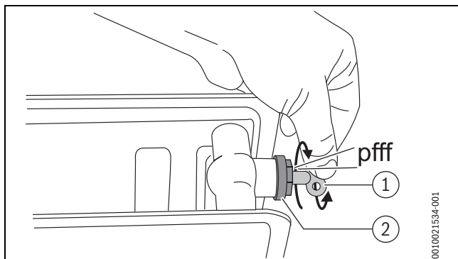
Bild 13 Heizkörper entlüften
