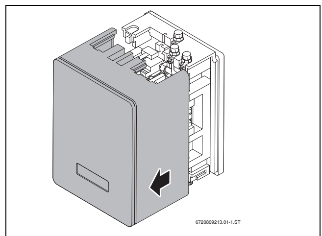
Bild 1 Station öffnen
