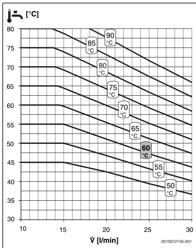
Bild 40 Temperaturverhalten FS20/2
