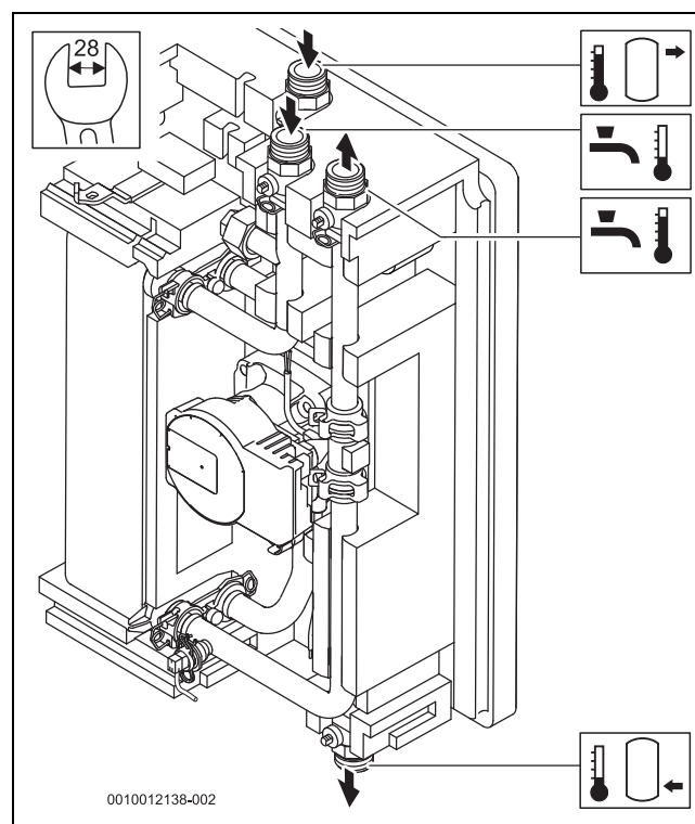
Bild 25 Anschlüsse Frischwasserstation
