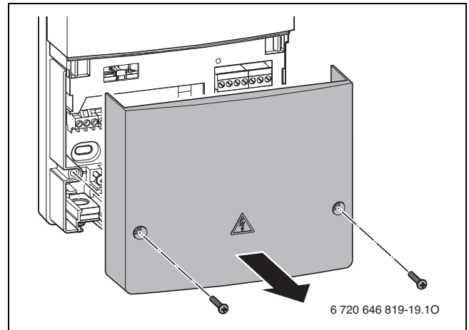
Bild 32 Modul öffnen
