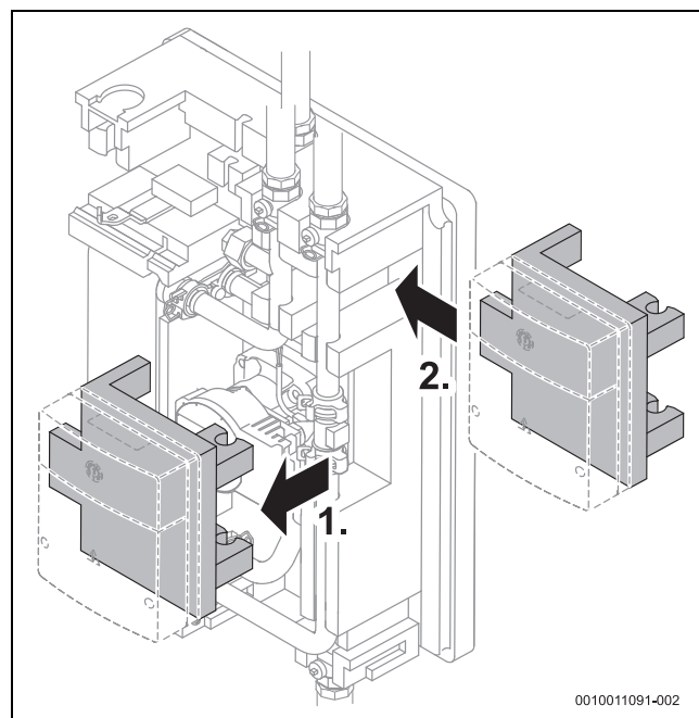
Bild 42 Modul für Wartungszwecke umstecken
