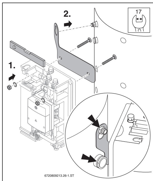
Bild 14 Halteblech montieren
