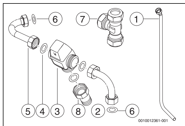
Bild 18 Lieferumfang Mischventil-Set
