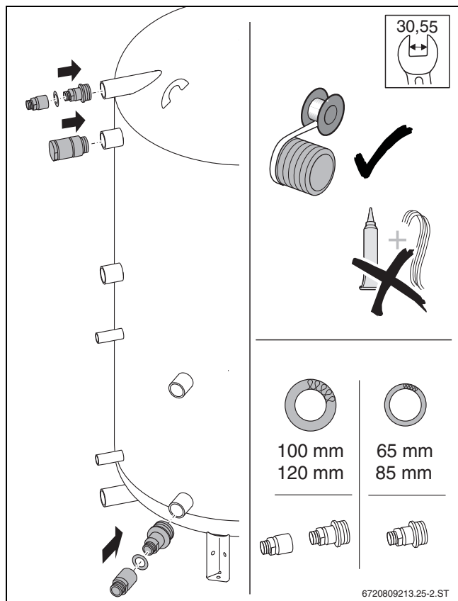
Bild 12 Anschlussstücke einschrauben
