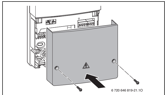
Bild 37 Abdeckung montieren
