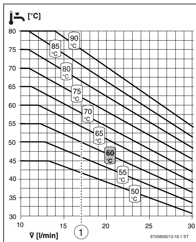
Bild 39 Temperaturverhalten FS/2
