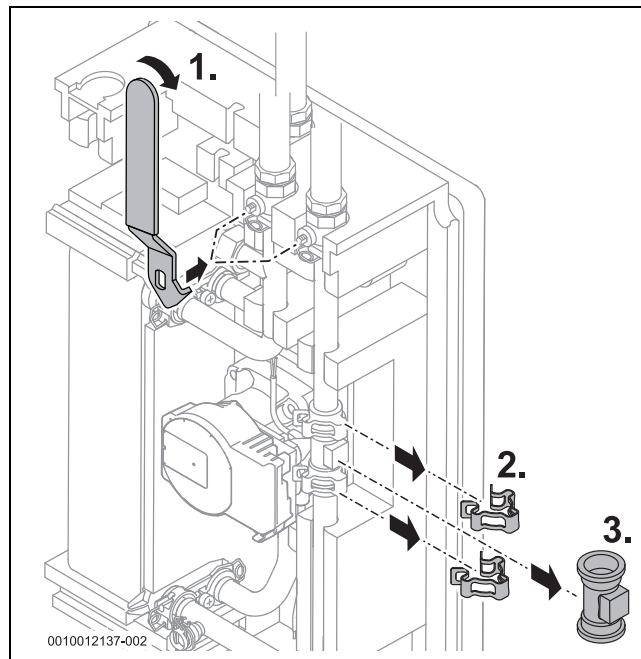
Bild 44 Volumenstromfühler demontieren
